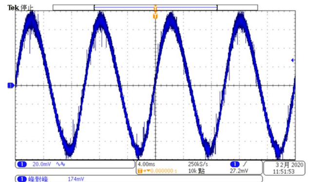
图 6: 出输出电压纹波与噪声(满载). (典型输入, 于输出端加 1uF MLCC 陶瓷电容)
