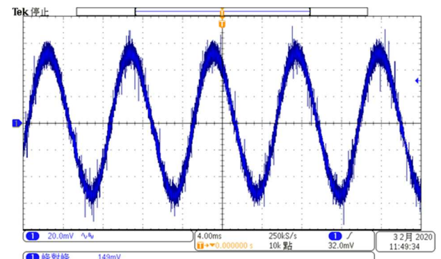
图 8: 出输出电压纹波与噪声(满载). (输入电压: 115V, 于输出端加 1uF MLCC 陶瓷电容)
